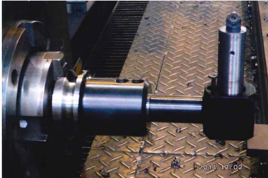
① ツール形状 Φ220～Φ260用
